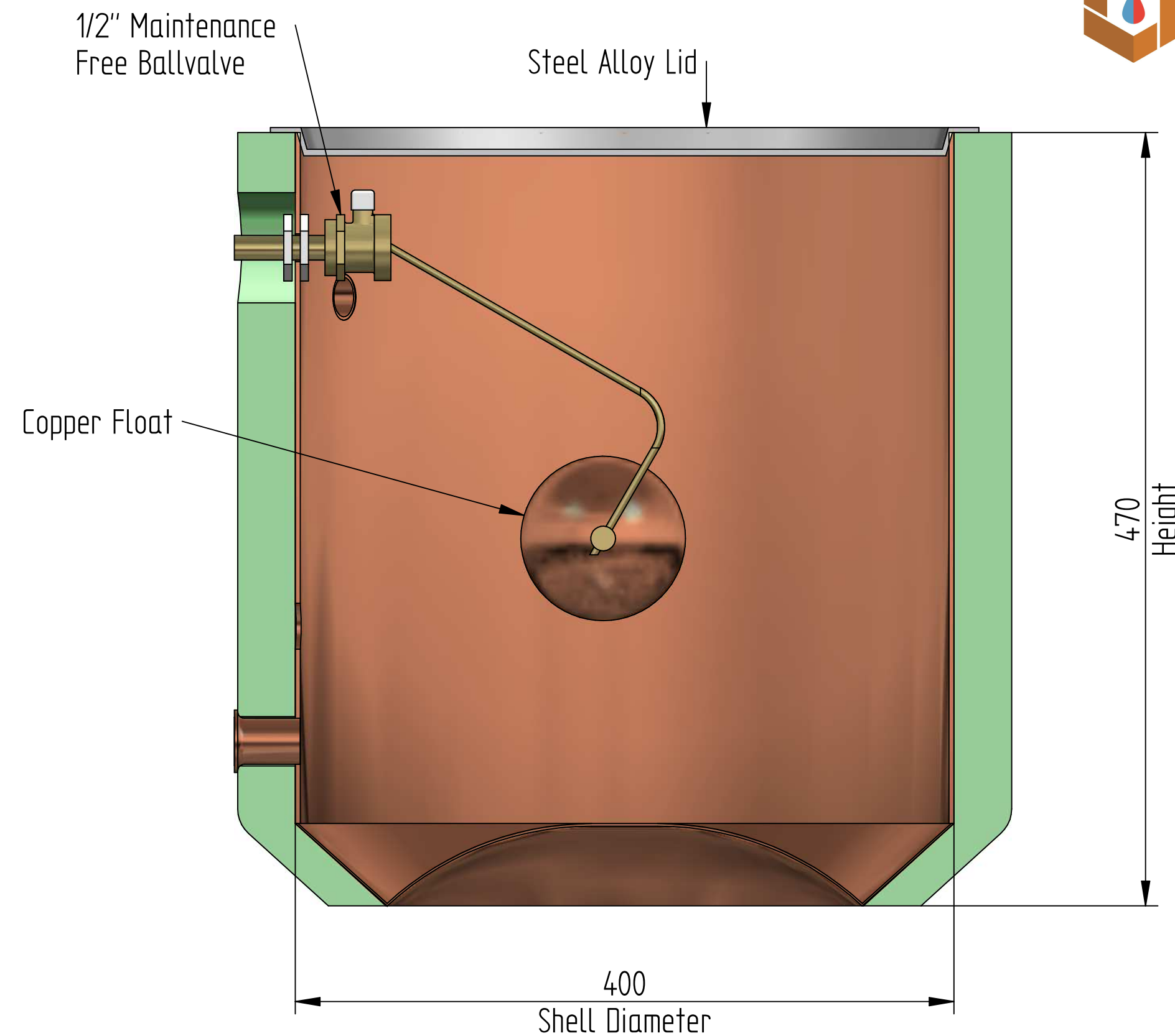
Section A-A
