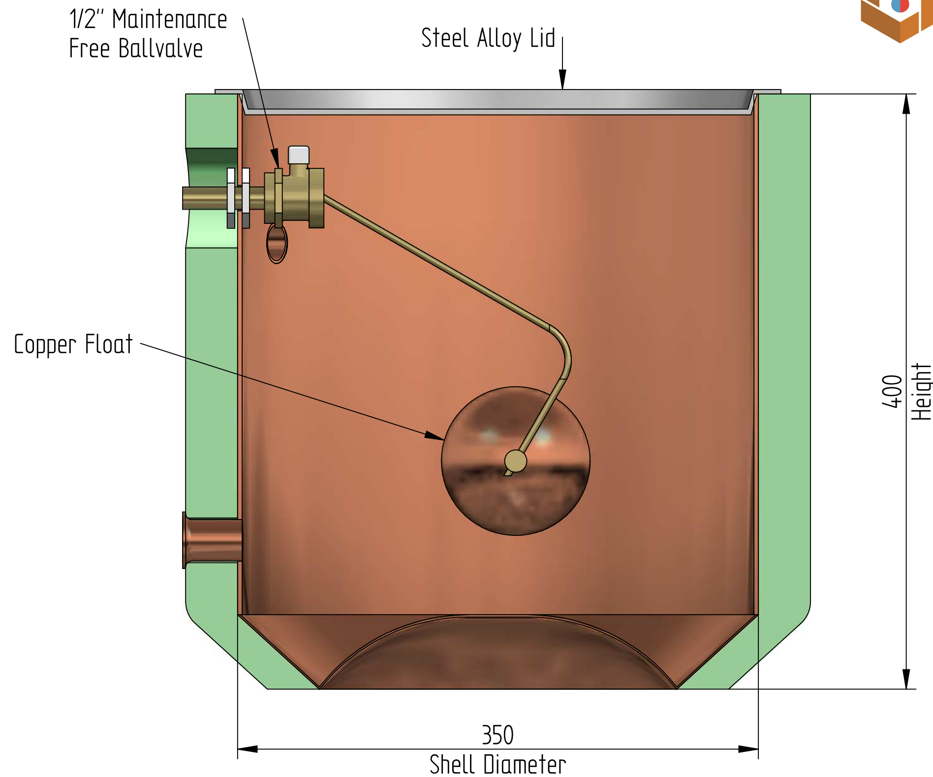
Section A-A
